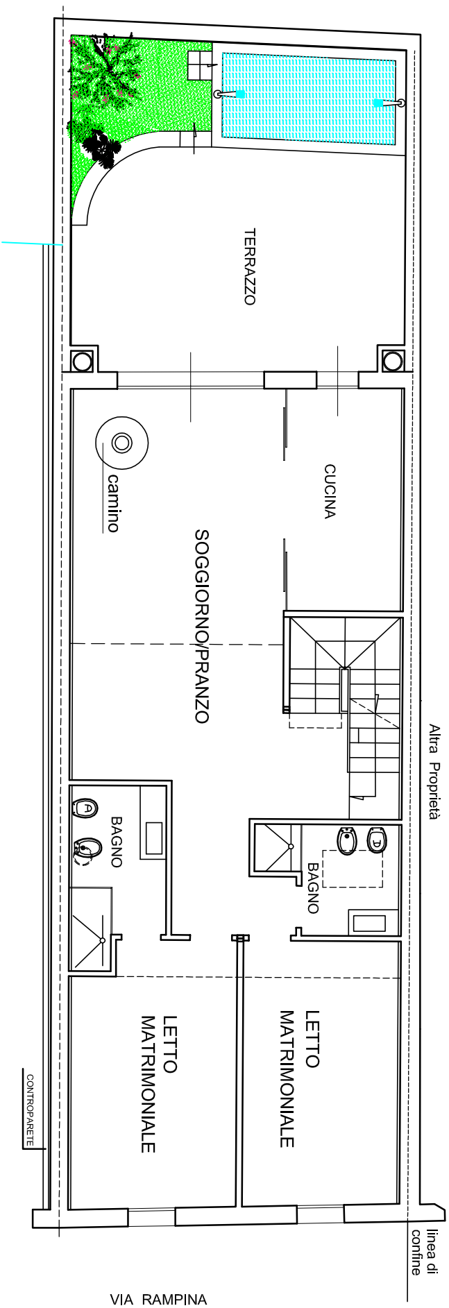
PIANTA PIANO PRIMO MQ. 123.85 Commerciali
